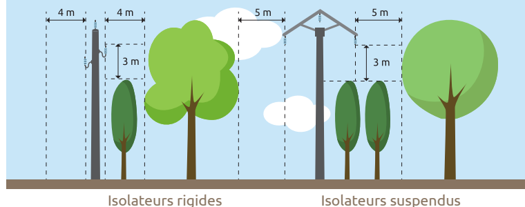
Isolateurs rigides
